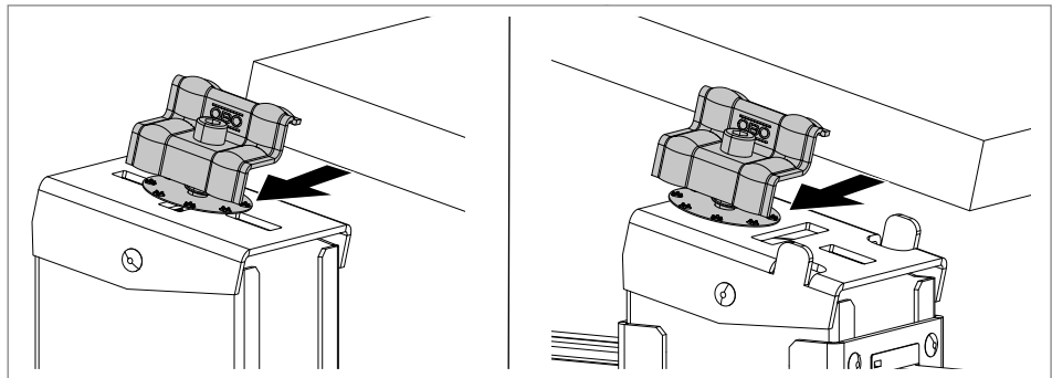
Jn. 25: Päikesepaneel lükata vastu otsaklambreid
