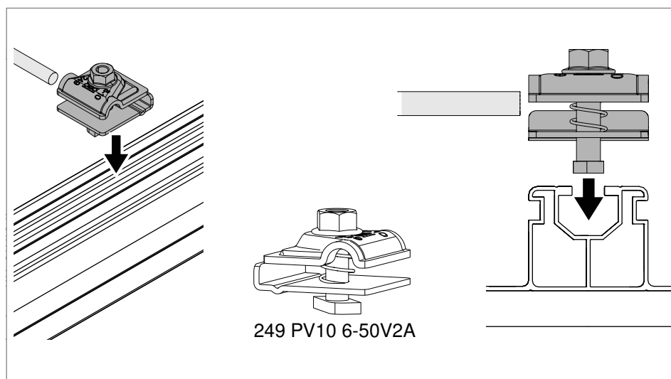
Jn. 40: Universaalse maandusklambri sisestamine kandeprofiili
