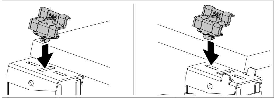
Jn. 24: Asetage otsaklambrid piludesse
