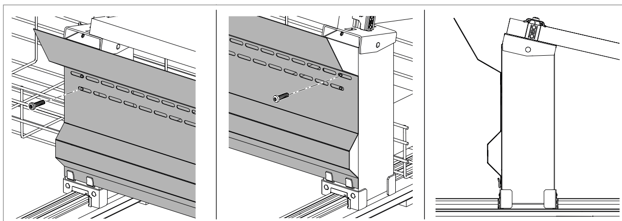
Jn. 39: Kruvige tuulekaitseplekk kinni
