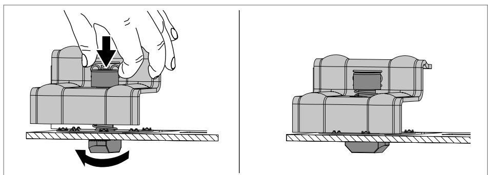
Jn. 26: Liugmutri lukustamine
