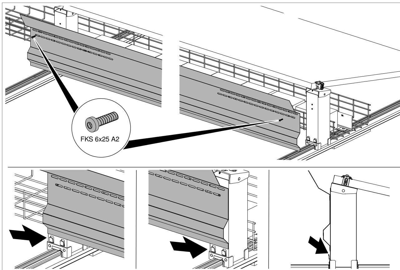
Jn. 38: Tuulekaitsepleki kinnitamine
